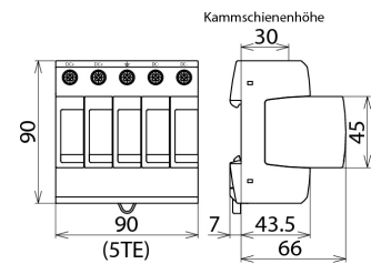
Maßbild DG M PV2 SCI 1000
