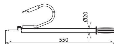
Maßbild EV TES 465 KS10
