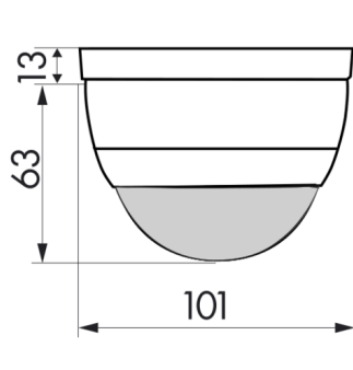
Bemaßung 92140
