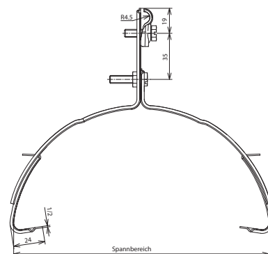
Maßbild DLH DQ 6.10 FG200.280 CU
