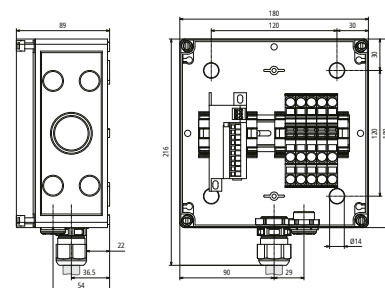
Maßbild DCU EMOB 2 32
