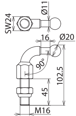
Maßbild KFP 20 W90 M16 45SSM
