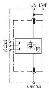
Prinzipialschaltbild DB M 1 320 FM
