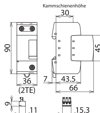
Maßbild DB M 1 320 FM
