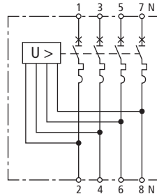
Prinzipschaltbild POP 4 255 C40
