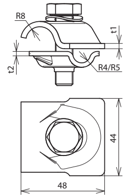
Maßbild MVK 8.10 16 SKM10X40 FSC V2A
