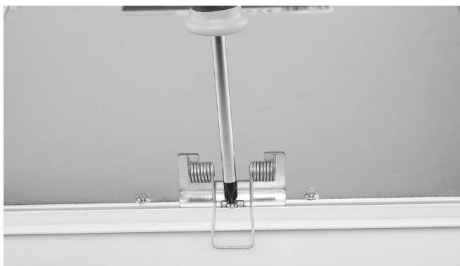
Abb. 7: SNAP-IN Federbügel für LED Panel SNAP Frame-In-One
