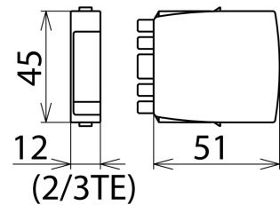
Maßbild BXT ML4 BD 180
