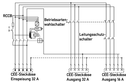
Anschlusschema
