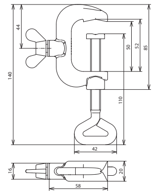
Maßbild EK 4.45 AQ6 16 TGTZN
