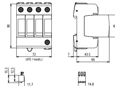
Maßbild DG MD TNS 275 FM
