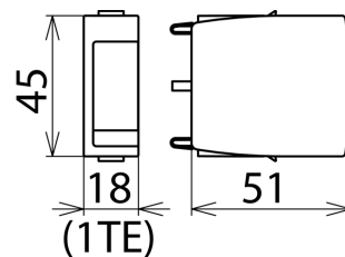
Maßbild DG MOD H PV 600
