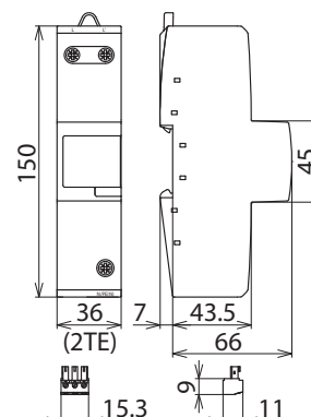
Maßbild DBM 1 760 FM
