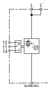
Prinzipialschaltbild DBM 1 760 FM
