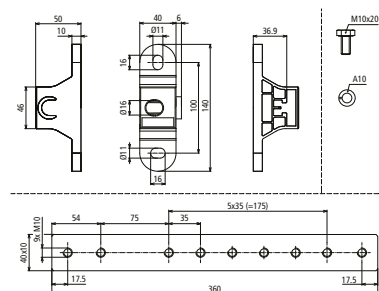
Maßbild PAS EX 7AP M10 V2A
