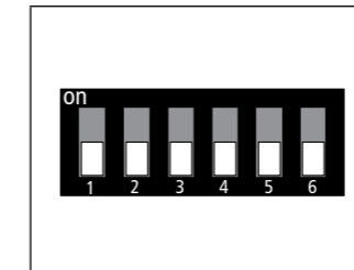
Abb. 07 DIP-Schalter
