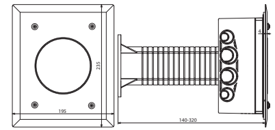
Maßbild TSKS WDVS 185X140X88 AH50.200
