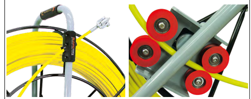
automatische Auslaufbremse Schnellauslauf mit gelagerten Laufrollen
