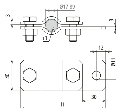
Maßbild ERS 76 AB11 STTZN
