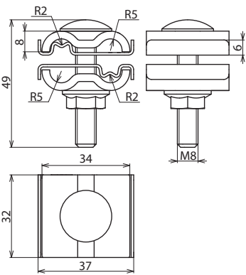
Maßbild UEK 8.10 AQ3/4 M8 V4A
