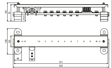
Maßbild
