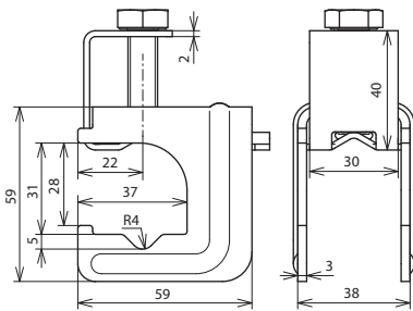
Maßbild VK DB 6.20 8.10 FL30 BSB STBL
