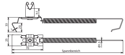
Maßbild DLH SGL 8 H32 FG180.280 V2A
