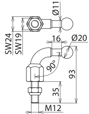
Maßbild KFP 20 W90 M12 35SSM
