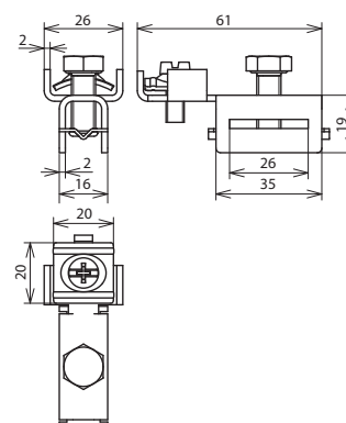
Maßbild SPK 25 BRS AQ4 25 V2A
