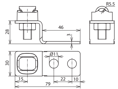
Maßbild ES ZF 2XB11 KSV 7.10 STTZN
