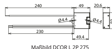
Maßbild DCOR L 2P 275
