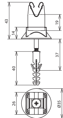
Maßbild LH DG 8 H20 HS5X50 KD8 V2A GR
