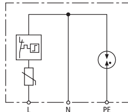
Prinzipschaltbild
