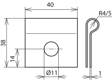
Maßbild KS 8 B11 STTZN
