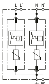
Prinzipschaltbild DG MP TN 275
