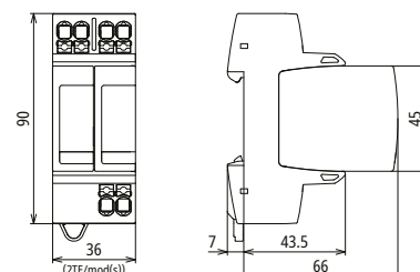
Maßbild DG MP TN 275
