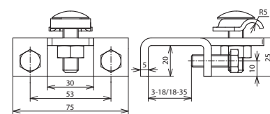
Maßbild AK 6.10 KB W KBF3 18 V2A
