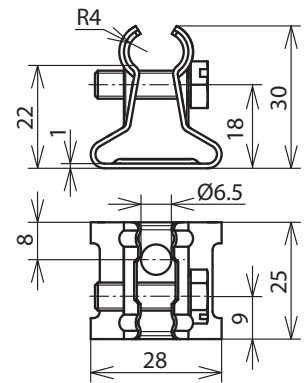
Maßbild LH KR 6.10 H22 B6.5 V2A
