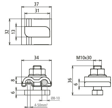
Maßbild UEK 8.10 AQ4 50 HKSBM10 V2A
