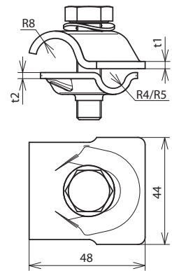
Maßbild MVK 8.10 16 SKM10X40 FSC STTZN
