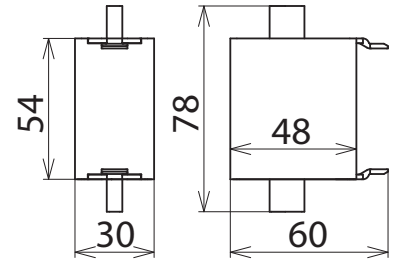
Maßbild
