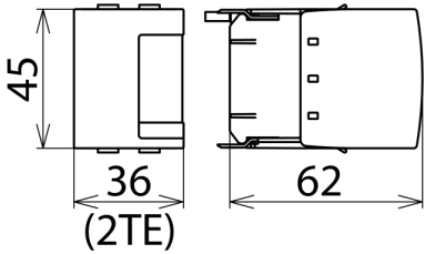
Maßbild DSE MOD 242
