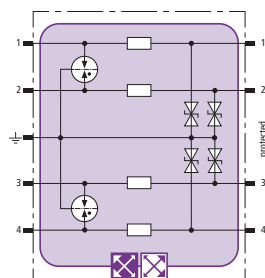
Prinzipschaltbild BXT ML4 BE 5
