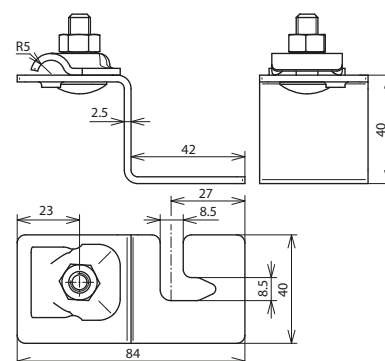
Maßbild DLH KB 6.10 TD B8.5 V2A
