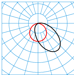
Sanesca W3 LED5000-840 01 (reading light) TX055770 ■ C0 - C180 ■ C90 - C270 DIN 5040: A30 UTE: 0,98 E + 0,02 T CEN Flux Code: 43 75 93 98 100 9 22 30 2
