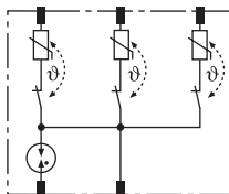
Prinzipschaltbild DR MOD 4P 255 SN1871
