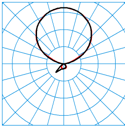
LuceoS S-U SMC PAW-IL 300-830 ETDI 03 (LEO2) TX369925 ■ C0 - C180 ■ C90 - C270 DIN 5040: E03 UTE: 0,08 D + 0,91 T CEN Flux Code: 53 86 96 8 100 49 82 98 92
