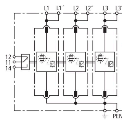
Prinzipialschaltbild DV M TNC 255 FM
