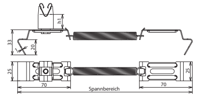
Maßbild DLH SG 8 H32 FG180.280 V2A
