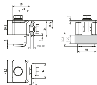
Maßbild AKK DUL 8.10 KBF 3 20 STTZN
