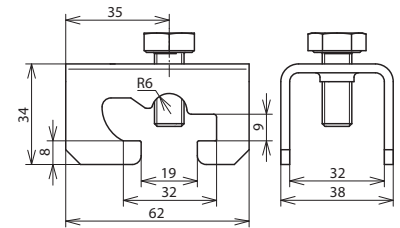
Maßbild VK EH R10 F30 ST
