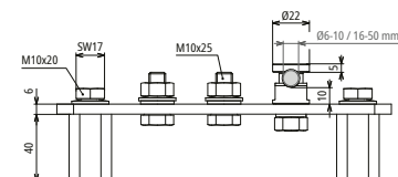
Maßbild PAS 3AP M10 KSM10 V4A
