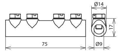
Maßbild VM 8 SKM6X10 ZG
